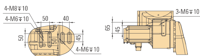
大臂孔位图 Lower arm
