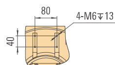
肩部孔位图 Shoulder arm
