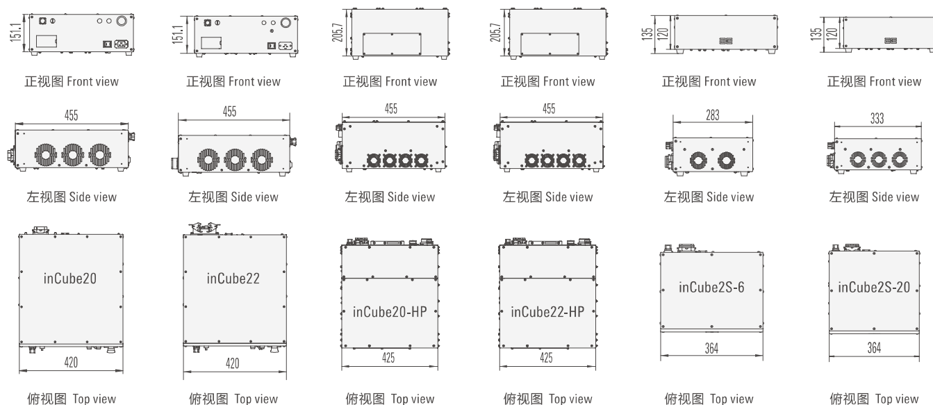
外形尺寸 Outline dimension
